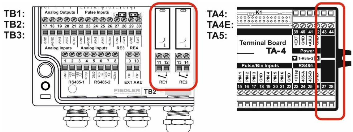
Umístění mechanických relé na přípojných deskách typu TB a TA
