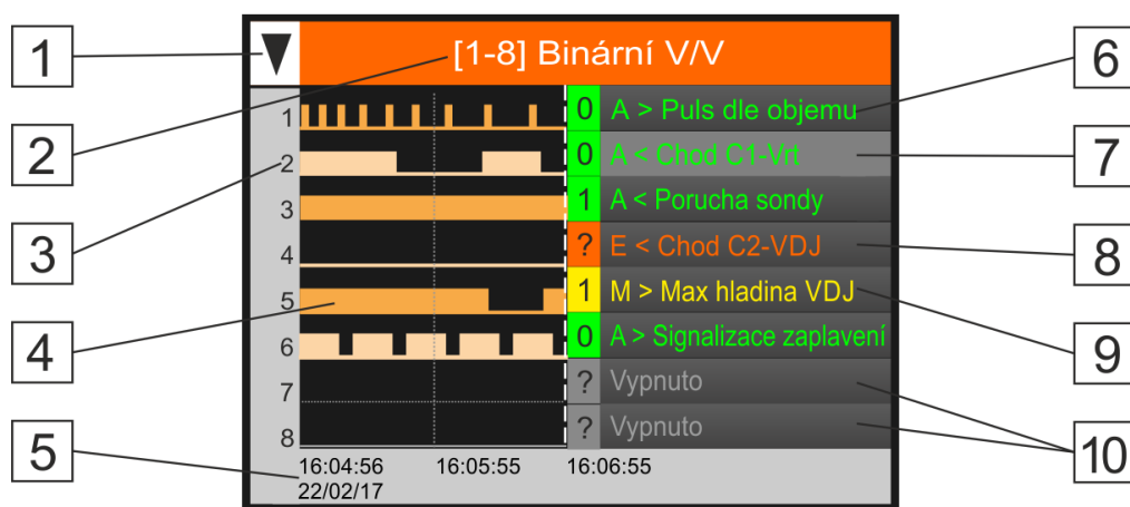
Obrazovka binárních kanálů
