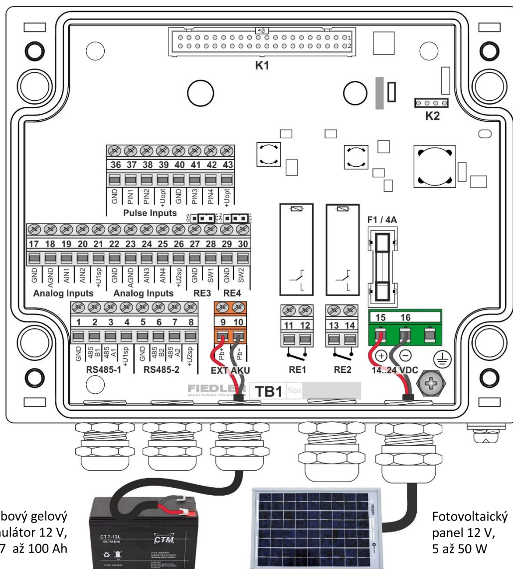
Zapojení svorek přípojné desky TB1
